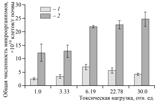
Рис. 1. Общая численность микроорганизмов в условиях химического загрязнения (1 – 2011 г., 2 – 2012 г.)
